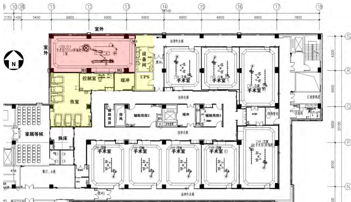
图 2-3 病房楼丁座六层 DSA 机房布局及周围环境示意图
