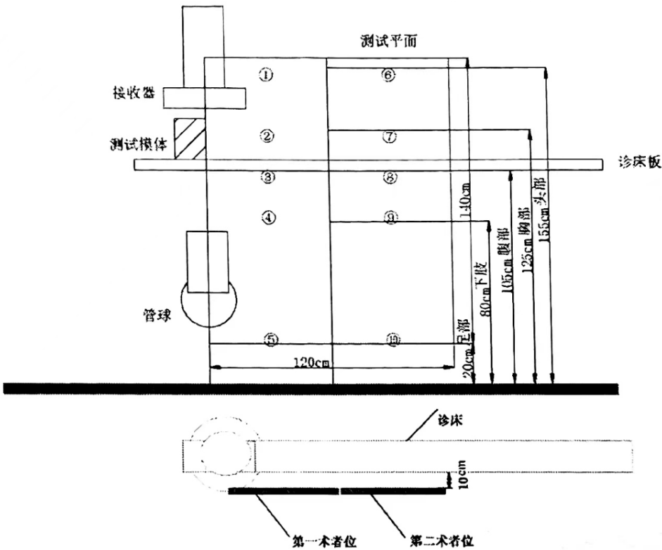
图 7-1 透视防护区测试点位示意图
